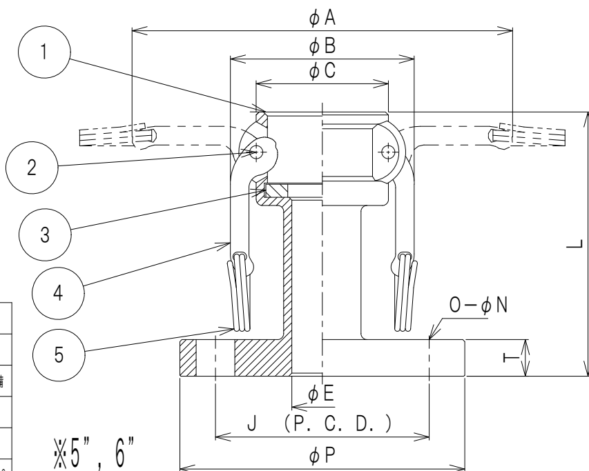
633-LBS SST サイズ別寸法表 (単位: mm)
